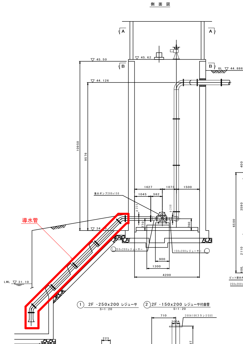
ポンプ配置図
