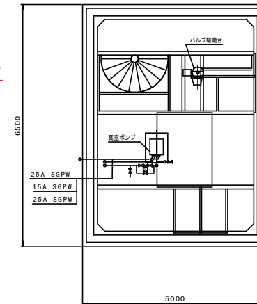
\underline{A - A}
