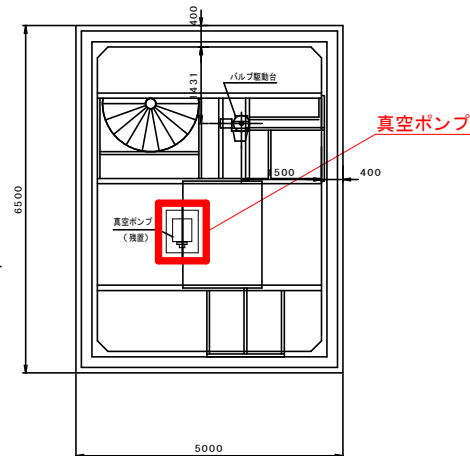
\underline{A - A}
